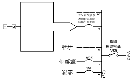
電路圖
